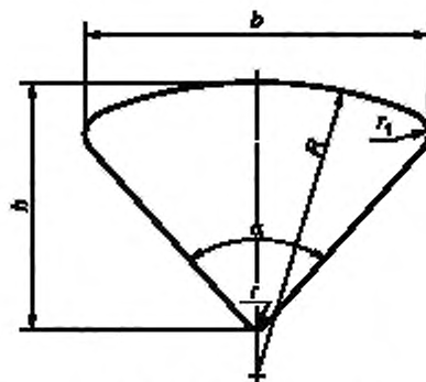
Рисунок А.2 — Конструкция секторных однопроволочных алюминиевых жил
